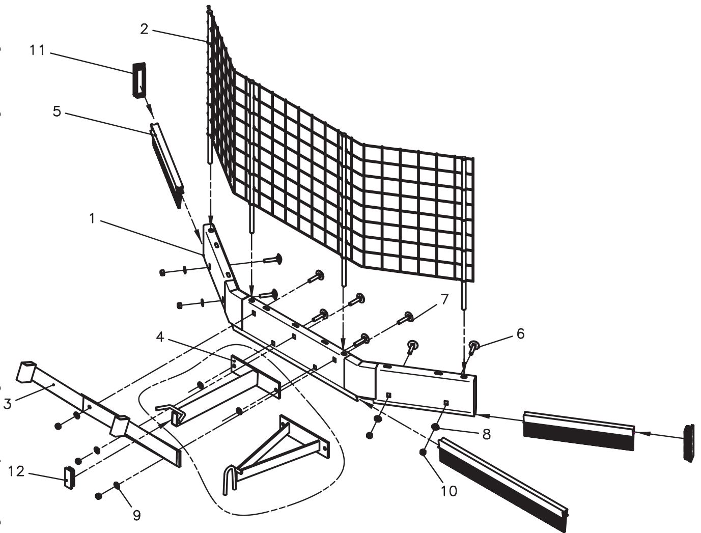
Explosionszeichnung
