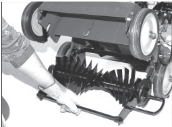
1) Feste Messer.
