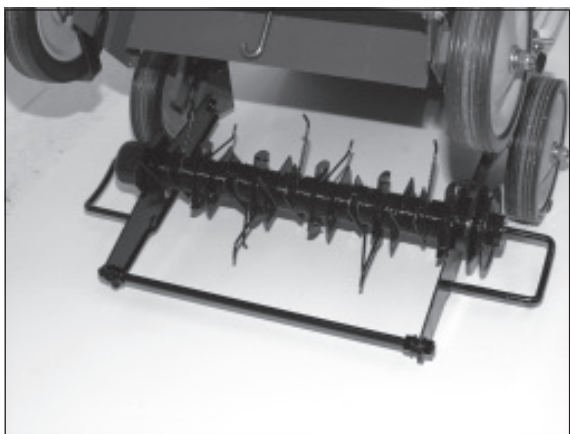
3) Federzinkenwelle
