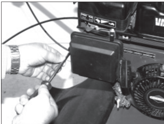
1) Schraube des Luftfilterdeckels lösen.
