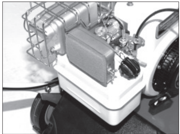
2) Deckel abnehmen.
