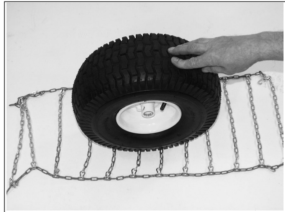
2) Demontiertes Rad auf die Schneekette stellen.
