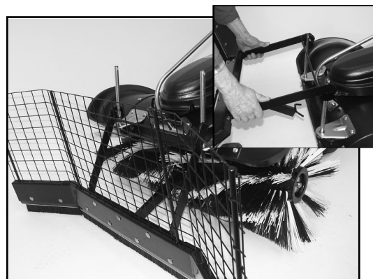
2) Den Laubsammler auf die Aufnahmestangen stecken, anschließend das Gitter aufsetzen.
