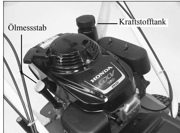
1) Kraftstoff- und Öltank beim Honda-Motor
