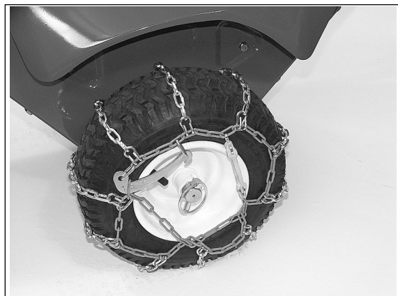
4) Das Rad mit montierter Schneekette auf die Achse stecken und anschließend mit dem Klappsplint sichern. Die zweite Kette auf die gleiche Weise montieren.
