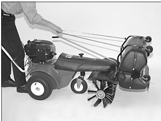
1) Um den Sammelbehälter zu entleeren, einfach vom Bedienerplatz aus am Zugbügel ziehen.
