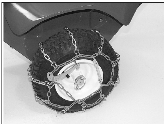
5) Das Rad mit montierter Schneekette auf die Achse stecken und anschließend mit dem Klappsplint sichern. Die zweite Kette auf die gleiche Weise montieren.
