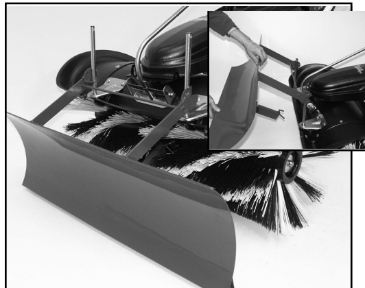
2) Das Räumschild auf die Aufnahmestangen stecken.
