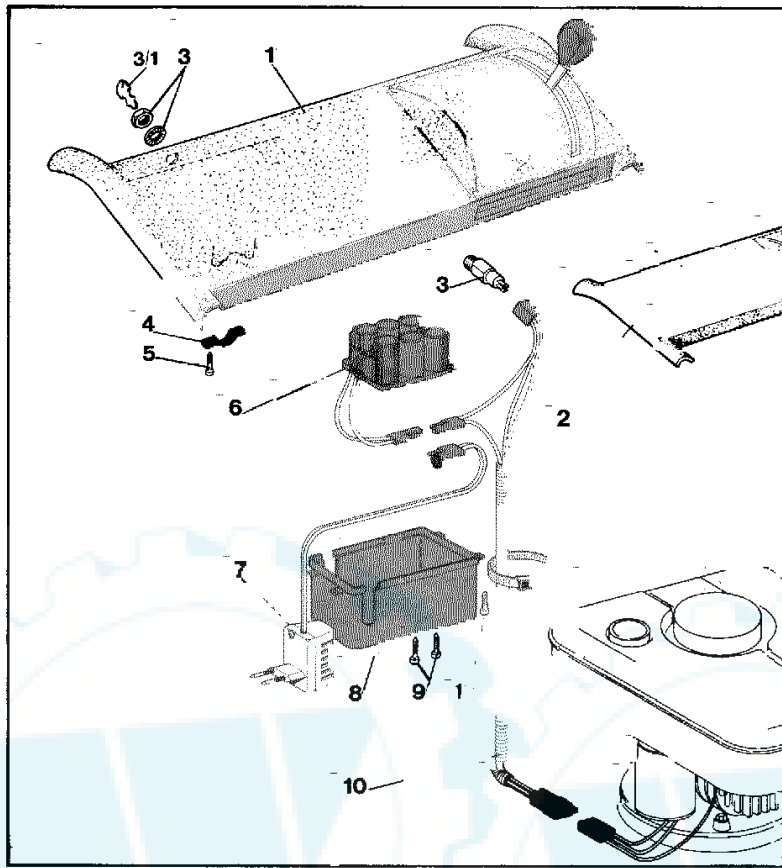
KIT AVVIAMENTO ELETTRICO mod. 943/CV/K - mod. 943/CVS/K - mod. 948/CVS/K
