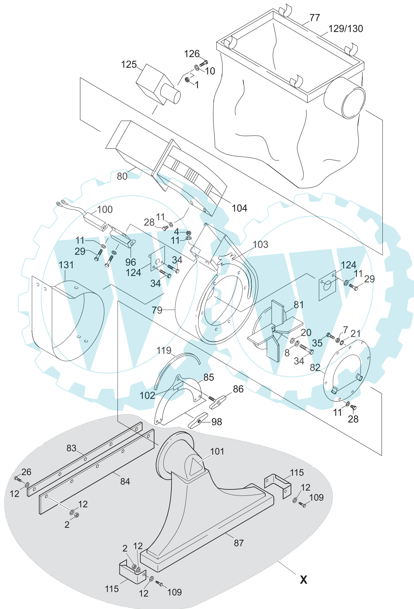
Turbine, Gehäuse, Fangsack Abb. 3
