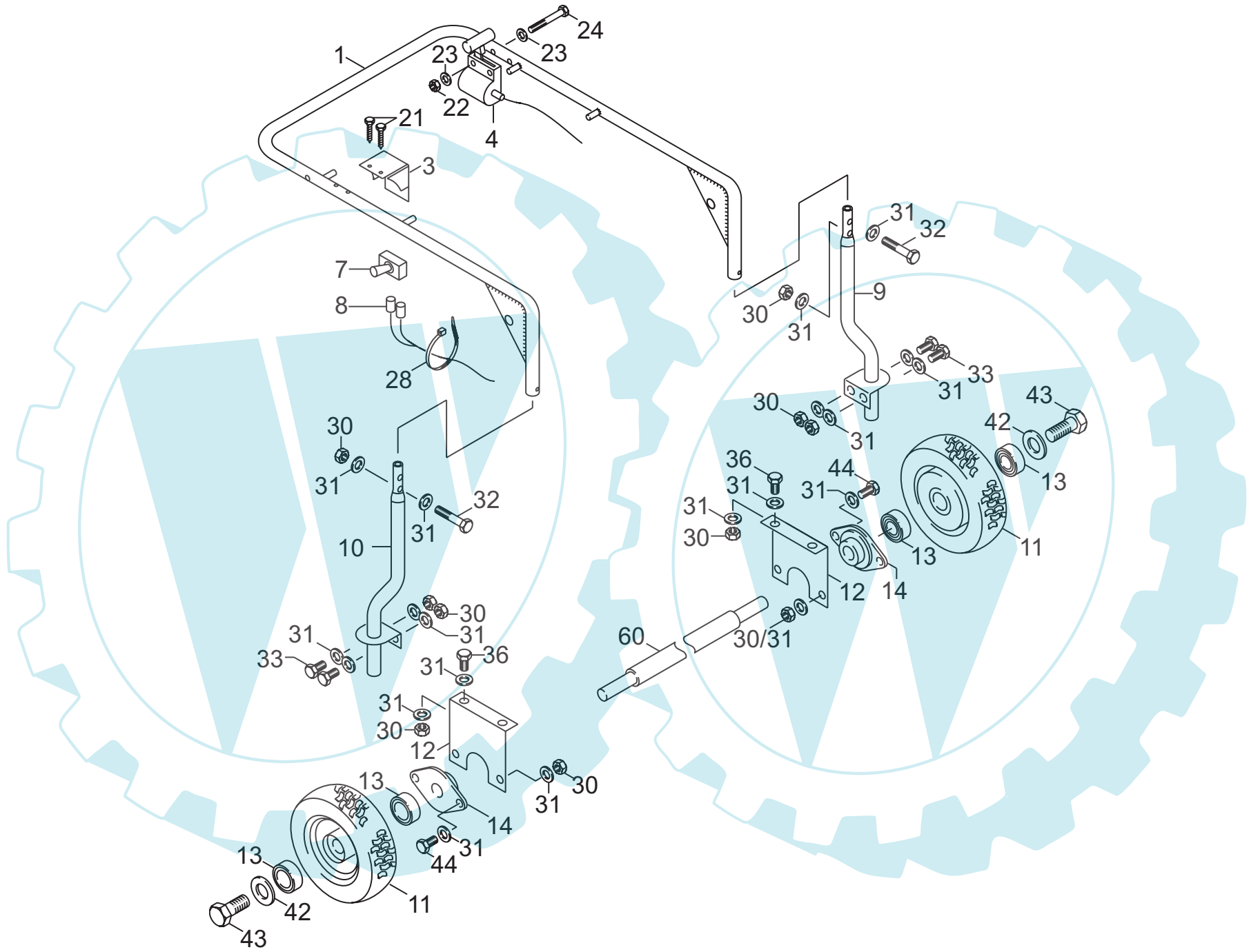
Führungsholm, Getriebe Abb. 1
