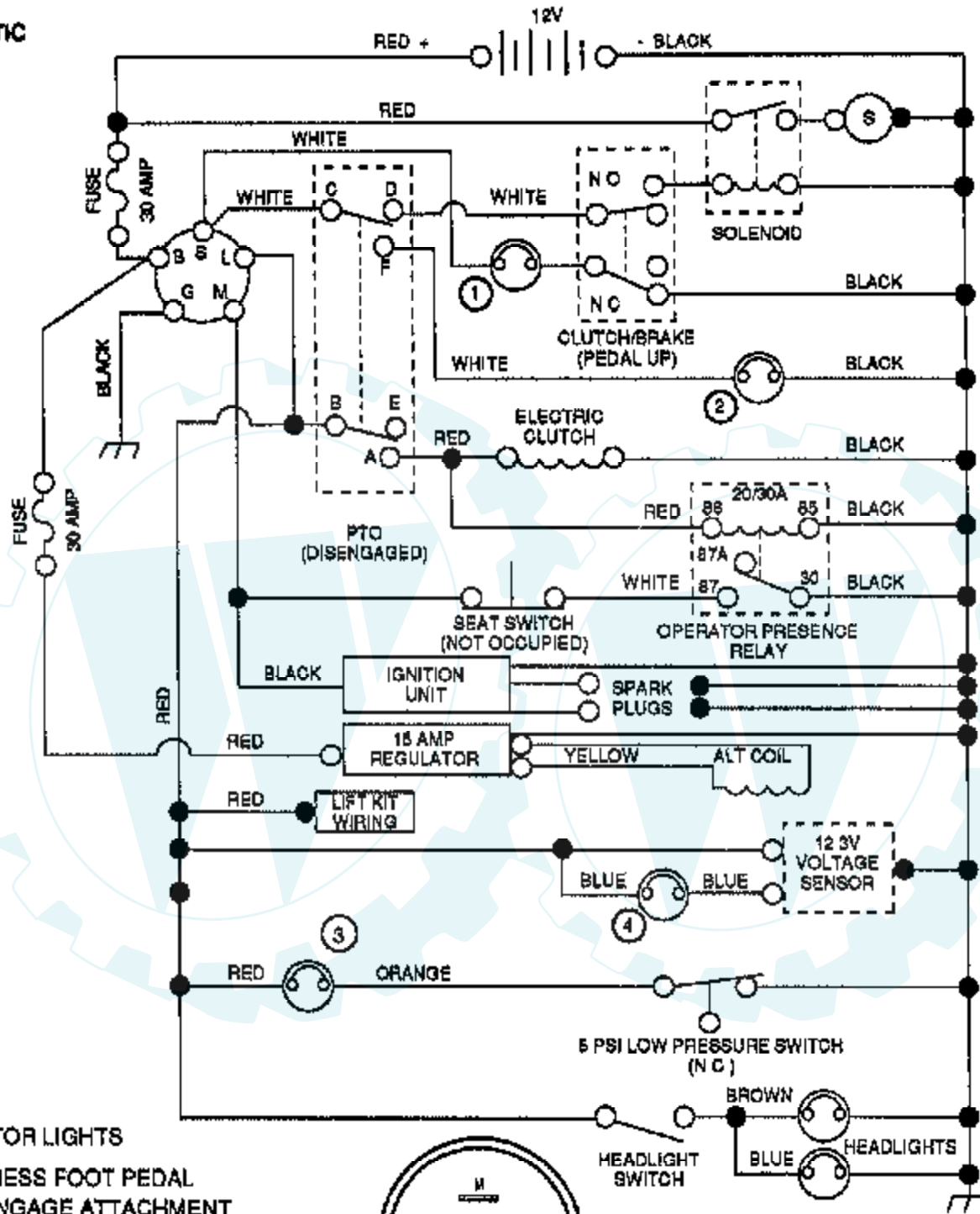
PTO SWITCH
